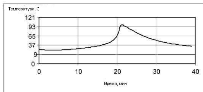
Стандартная экзотермическая кривая для MA320 при 23°C (10 грамм) 5
