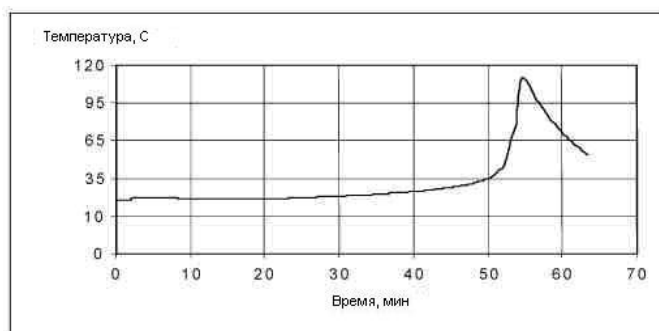
Стандартная экзотермическая кривая для MA550 при 23°C (10 грамм) 5
