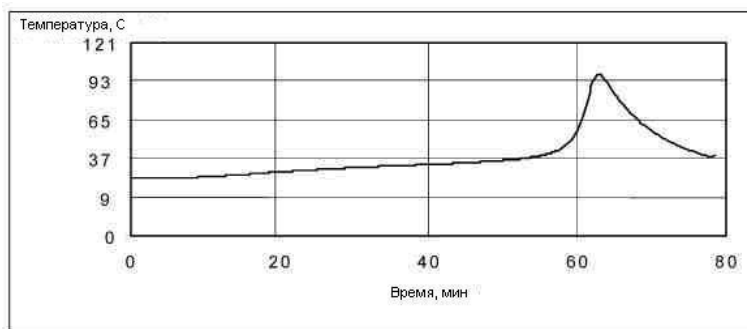
Стандартная экзотермическая кривая для MA425 при 23°C (10 грамм) 5
