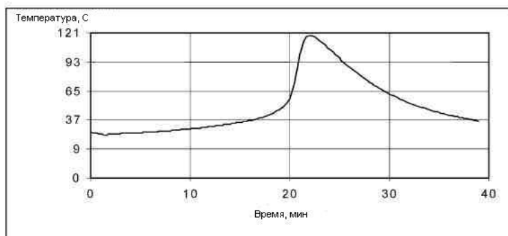
Стандартная экзотермическая кривая для MA310 при 23°C (10 грамм) 5
